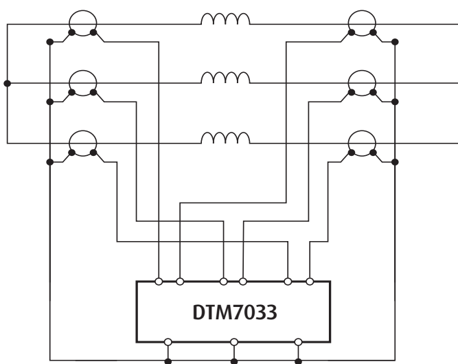
Figure 1 - Protection différentielle longitudinale de machine Machine longitudinal differential protection
