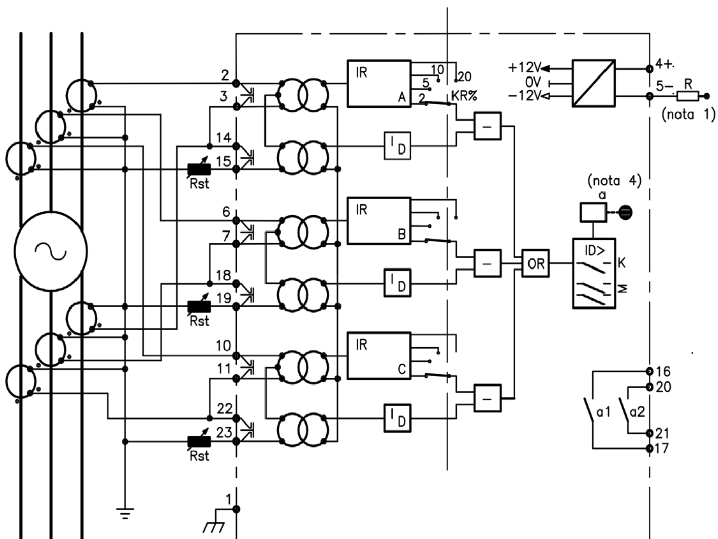
Figure 3 - Schéma de fonctionnement simplifié et de raccordement Simplified operating and connection diagram
