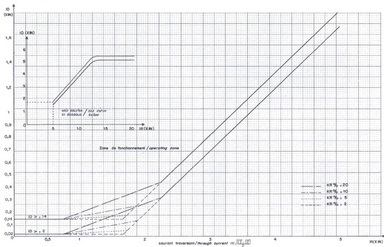
Figure 4 - DTM7033 - Courbes de fonctionnement / Operating characteristics
