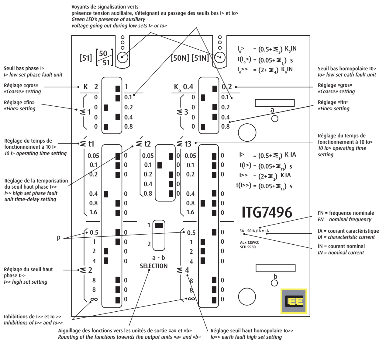
Figure 1 Face avant relais ITG7496 / ITG7496 relay front-plate Modèle bi ou triphasé + homopolaire à temps extrêmement inverse et avec seuils hauts Two or three-phase + earth fault unit model extremely inverse time and with high set units.
