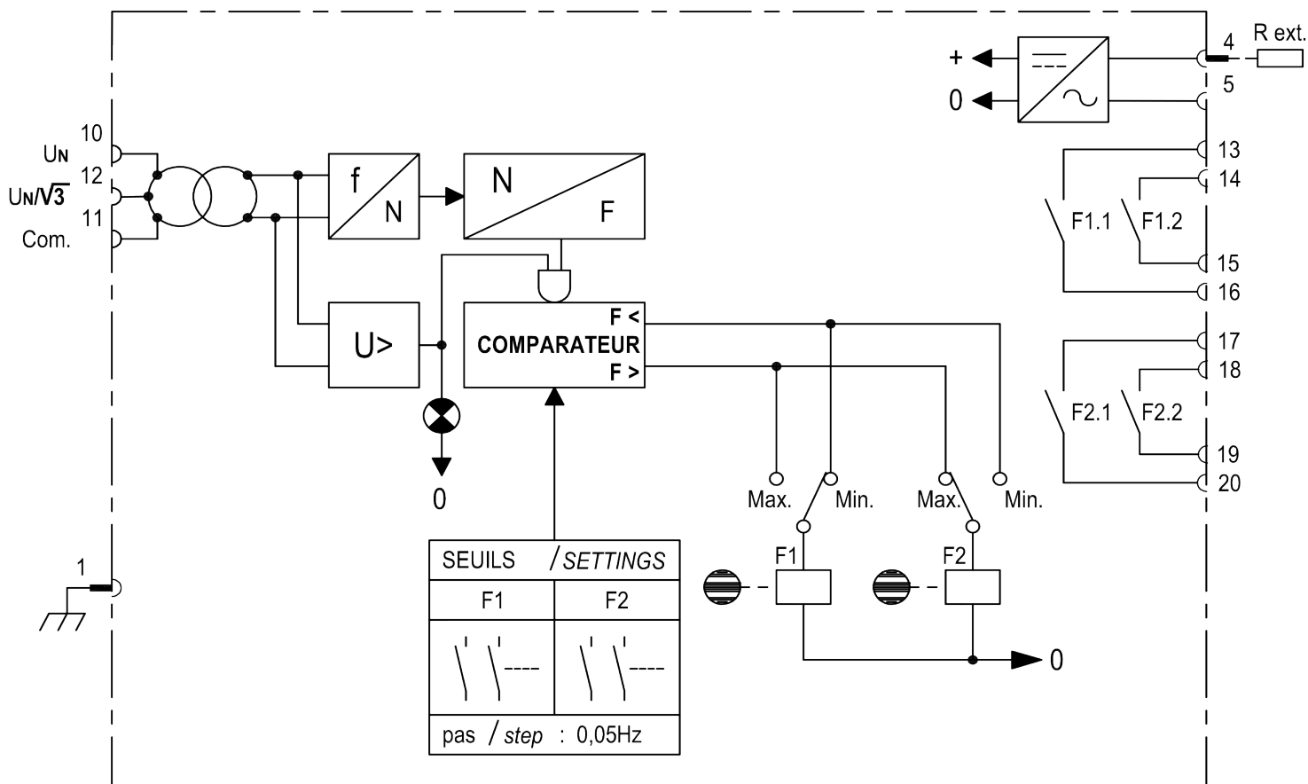
HDG7020 - Schéma de fonctionnement et de raccordement simplifié Simplified operation and connection diagram
