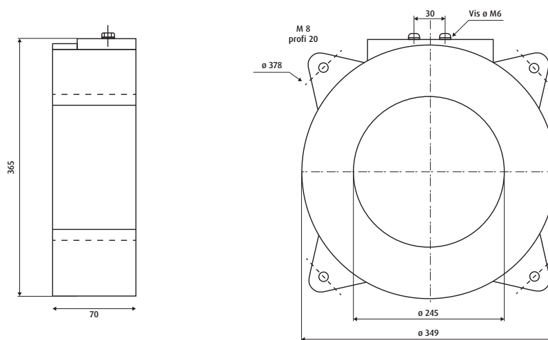
Encombrement TC tore TF 245-1 ou TF 245-15
