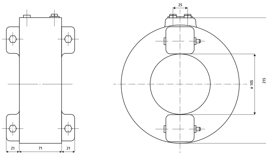
Encombrement TC tore TO 105-1 ou TO 105-15
